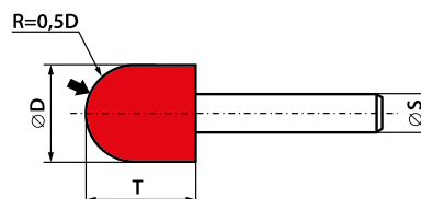
SPOSÓB OZNACZANIA 5213 - D × T × S
