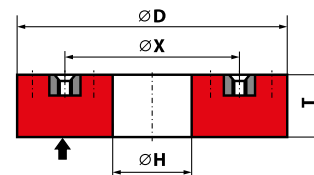
36 - D \times T \times H - ... - nr rysunku
