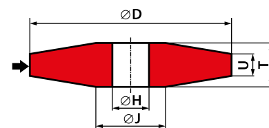
SPOSÓB OZNACZANIA 4 - D/J × T/U × H
