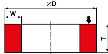
SPOSÓB OZNACZANIA 2 - D × T - W...
