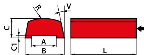
SPOSÓB OZNACZANIA 3113 - B/A × C × L - R...V...
