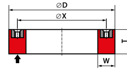
Typ 37 Ściernica pierścieniowa z wkładkami gwintowymi 37 - D \times T - W... - nr rys.
