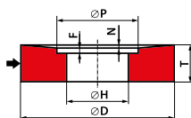
Typ 23 Ściernica z jednostronnym wybraniem stożkowo - walcowym 23 - D \times T/N \times H - P... F...
