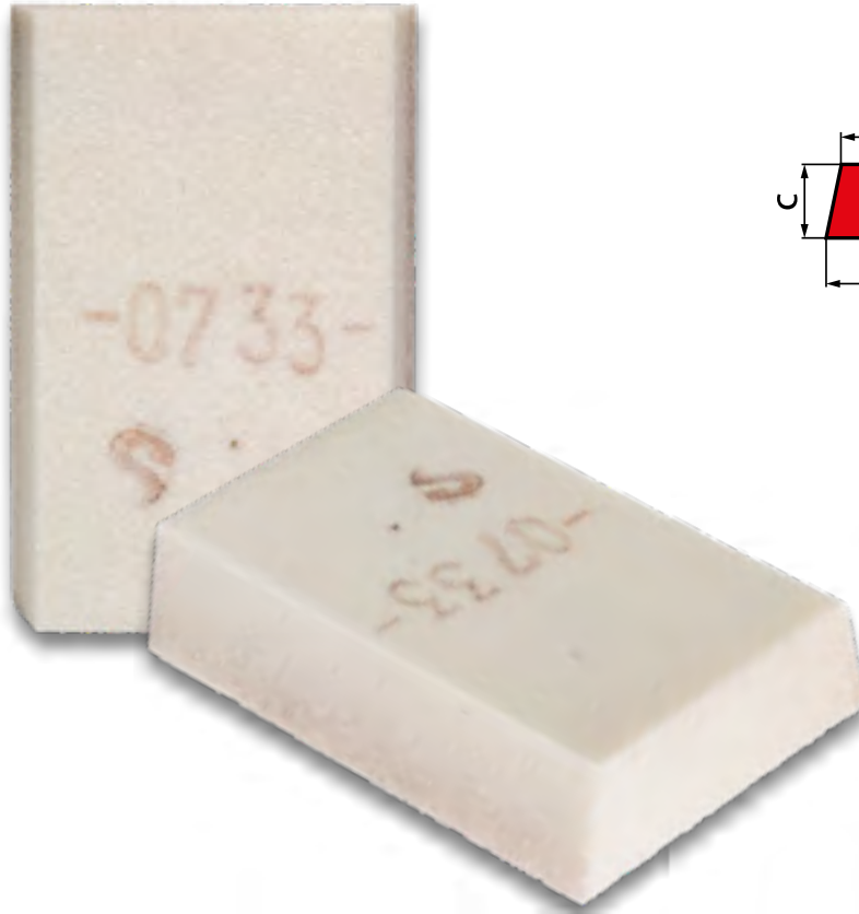
SPOSÓB OZNACZANIA 3109 - B/A × C × L
