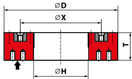
3601 - D × T × H - nr rysunku
