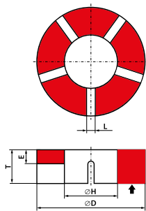
Typ 3501 Ściernica tarczowa z nacięciami 3501 - D \times T / E \times H - L...n - n - \text{ilość nacięć}
