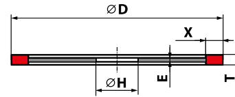
SPOSÓB OZNACZANIA 1A1R - D × T × X × E × H
