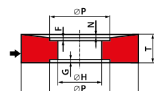
Typ 24 Ściernica z wybraniem stożkowo - walcowym i walcowym z drugiej strony 24 - D \times T/N \times H - P... F... G...
