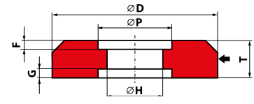
7X - D × T × H - P...F...G... - nr rysunku
