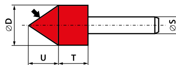
SPOSÓB OZNACZANIA 5211 - D × T × S - V
