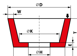
SPOSÓB OZNACZANIA 11 - D/J × T × H - W...E...K...
