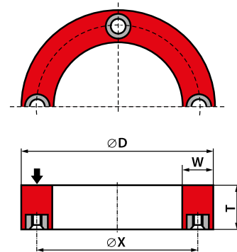
SPOSÓB OZNACZANIA 37 - D × T - W - nr rysunku W < 0,17D
