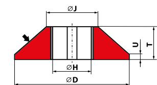
301X - D/J × T/U × H - nr rysunku
