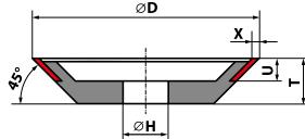
Typ 12V9 Ściernica diamentowa i borazonowa 12V9 - D × T × X × U × H
