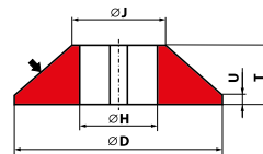
Typ 301 Ściernica do obtuskiwaczy ziarna EKONOS 301 - D / J × T / U × H
