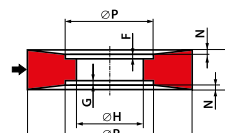
Typ 26 Ściernica z dwustronnym wybraniem stożkowo - walcowym 26 - D \times T/N \times H - P... F... G...
