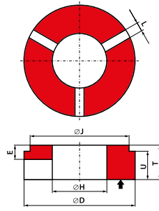
Typ 3504 Ściernica tarczowa z nacięciami jednostronnie odsadzona 3504 - D / J \times T / U / E \times H - L...n - n - \text{ilość nacięć}
